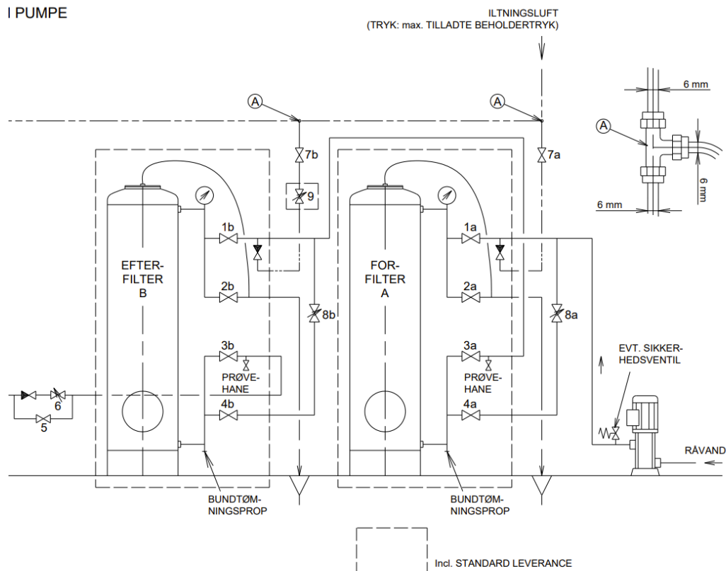
Figur 1: Indretning af filtrene efter renoveringen.
