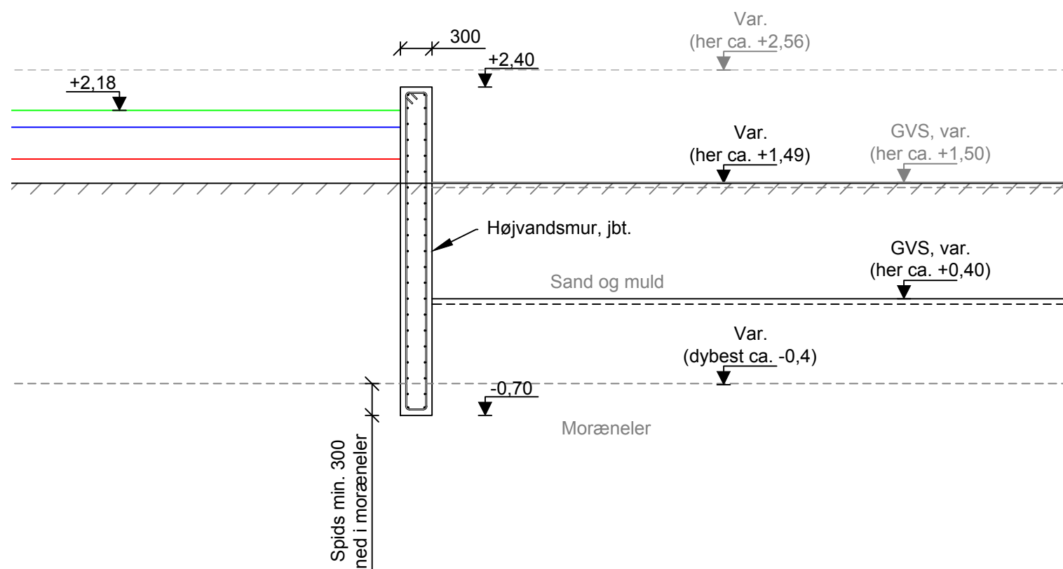
Principalsnit, 1:50
